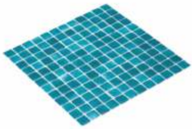
Ürün Kodu/Product Code HVZ-123 Plaka Ölçüsü/Sheet Size 31.5x31.5 cm Taş Ölçüsü/Chip Size 25x25 mm Kalınlık/Thickness 4.5 mm
