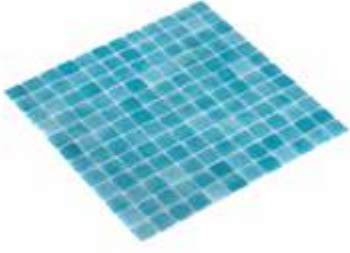
Ürün Kodu/Product Code HVZ-080 Plaka Ölçüsü/Sheet Size 31.5x31.5 cm Taş Ölçüsü/Chip Size 25x25 mm Kalinlık/Thickness 4.5 mm
