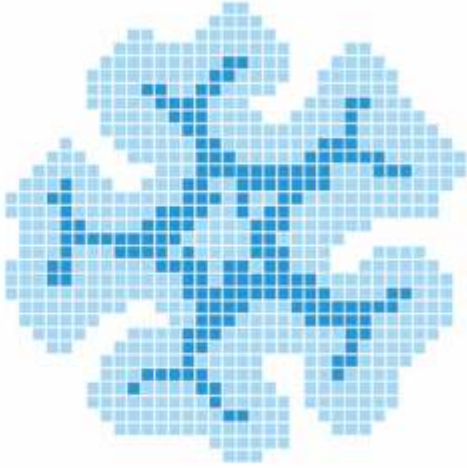
Ürün Kodu/Product Code HVZ-718 Taş Ölçüsü/Chip Size 25x25 mm Kalınlık/Thickness 4.5 mm Desen Ölçüsü/Pattern Size 95x95 cm
