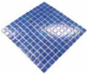
Ürün Kodu/Product Code HVZ-4125 Plaka Ölçüsü/Sheet Size 31.5x31.5 cm Taş Ölçüsü/Chip Size 25x25 mm Kalinlık/Thickness 4.5 mm
