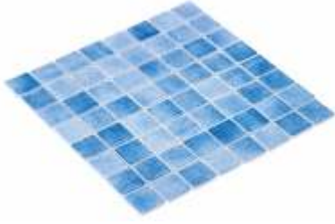
Ürün Kodu/Product Code HVZ-183 Plaka Ölçüsü/Sheet Size 31.5x31.5 cm Taş Ölçüsü/Chip Size 38x38 mm Kalinlık/Thickness 6.2 mm
