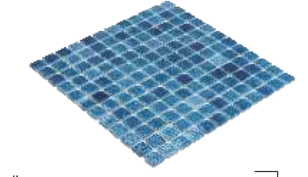
Ürün Kodu/Product Code HVZ-140 Plaka Ölçüsü/Sheet Size 31.5x31.5 cm Taş Ölçüsü/Chip Size 25x25 mm Kalinlık/Thickness 4.5 mm
