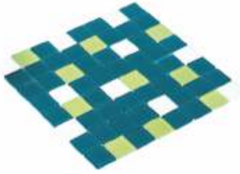
Ürün Kodu/Product Code HVZ-507 Plaka Ölçüsü/Sheet Size 31.5x31.5 cm Taş Ölçüsü/Chip Size 38x38 mm Kalınlık/Thickness 4 mm Flt
