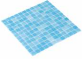
Ürün Kodu/Product Code HVZ-081 Plaka Ölçüsü/Sheet Size 31.5x31.5 cm Taş Ölçüsü/Chip Size 25x25 mm Kalinlık/Thickness 4.5 mm
