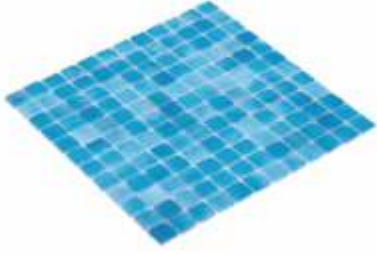
Ürün Kodu/Product Code HVZ-120 Plaka Ölçüsü/Sheet Size 31.5x31.5 cm Taş Ölçüsü/Chip Size 25x25 mm Kalınlık/Thickness 4.5 mm
