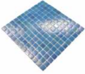
Ürün Kodu/Product Code HVZ-4111 Plaka Ölçüsü/Sheet Size 31.5x31.5 cm Taş Ölçüsü/Chip Size 25x25 mm Kalinlık/Thickness 4.5 mm
