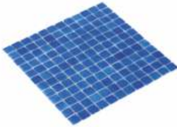
Ürün Kodu/Product Code HVZ-083 Plaka Ölçüsü/Sheet Size 31.5x31.5 cm Taş Ölçüsü/Chip Size 25x25 mm Kalinlık/Thickness 4.5 mm
