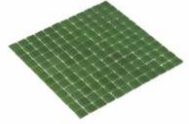
Ürün Kodu/Product Code HVZ-418 Plaka Ölçüsü/Sheet Size 30x30 cm Taş Ölçüsü/Chip Size 23x23 mm Kalinlık/Thickness 4 mm Flt
