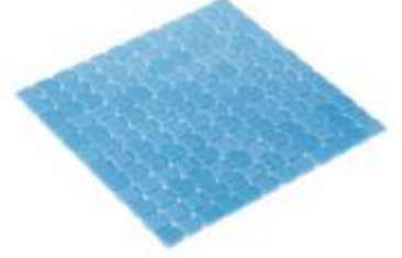
Ürün Kodu/Product Code HVZ-011 Plaka Ölçüsü/Sheet Size 31.5x31.5 cm Taş Ölçüsü/Chip Size 25x25 mm Kalınlık/Thickness 4.5 mm
