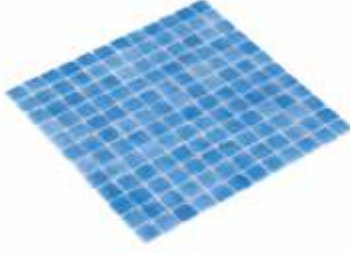
Ürün Kodu/Product Code HVZ-082 Plaka Ölçüsü/Sheet Size 31.5x31.5 cm Taş Ölçüsü/Chip Size 25x25 mm Kalinlık/Thickness 4.5 mm
