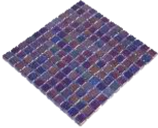
Ürün Kodu/Product Code HVZ-4116 Plaka Ölçüsü/Sheet Size 31.5x31.5 cm Taş Ölçüsü/Chip Size 25x25 mm Kalinlık/Thickness 4.5 mm
